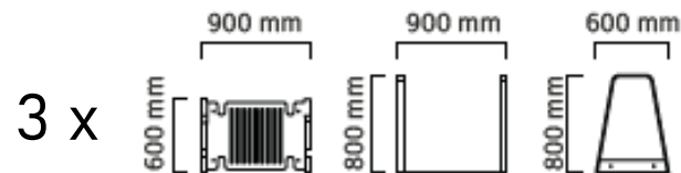
FAHRRADSTÄNDER - GROß
