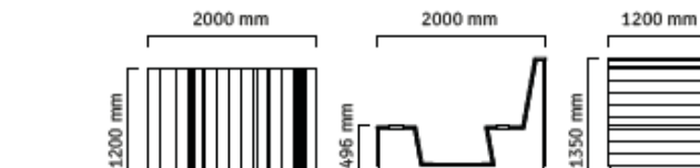
PARKLET-SITZMODUL
